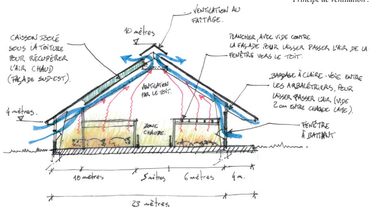
Principe de ventilation :
